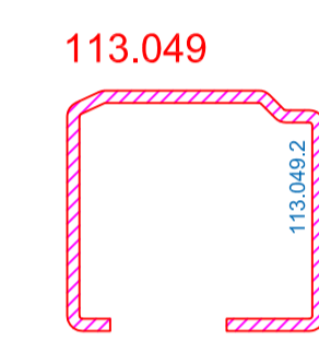
Створка 105mm / Артикул: 103.408 Усилитель: 113.049 Соединитель: 113.147
